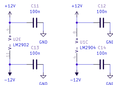
DECOUPLING CAPS
